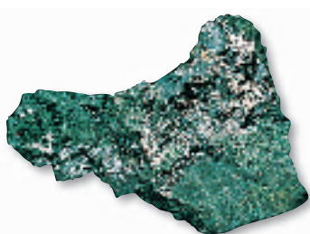
Ilmenite
